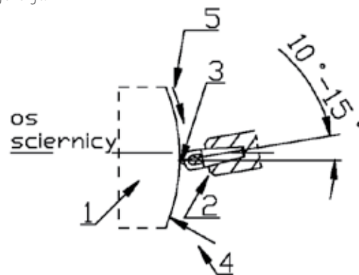
Abb. 1. Stellung des Abrichtdiamanten während des Abrichtens der Schleifscheibe 1 – Richtung des Längsvorschubs, 2 – Richtung der Drehbewegung der Schleifscheibe, 3 – Richtung der Tiefe des Abrichtens, 4 – Größe der einmalig abgerichteten Schicht, 5 – Fließrichtung der Kühlflüssigkeit.
